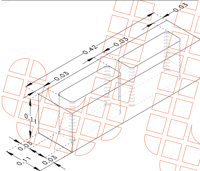
ISOMÉTRICO - Cotas en Metros
