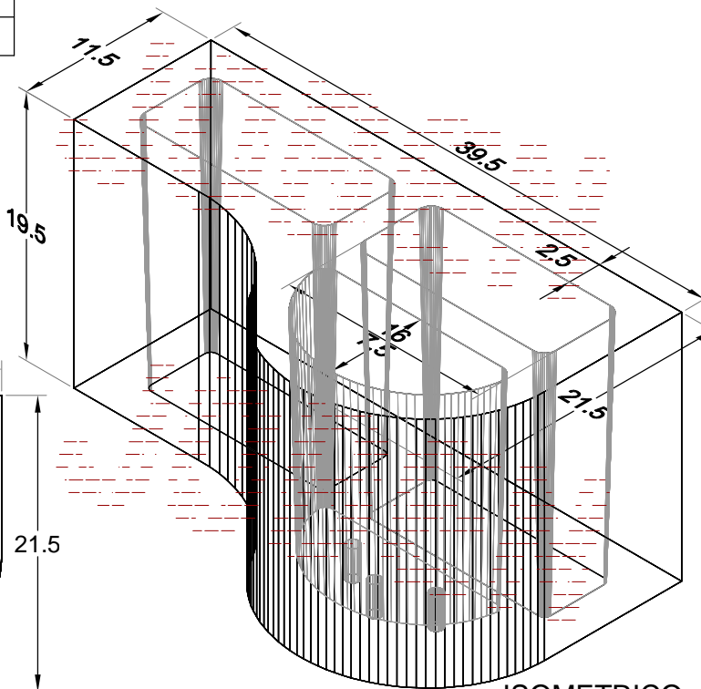
ISOMETRICO
